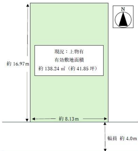
〈地形図〉
