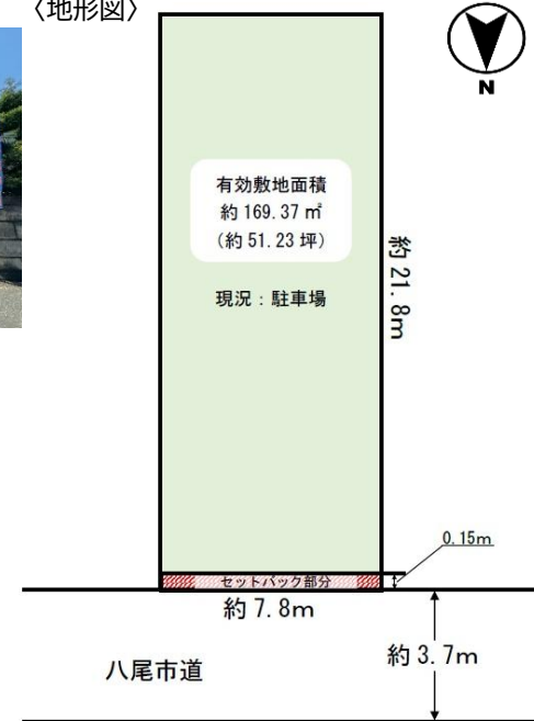
〈地形図〉
